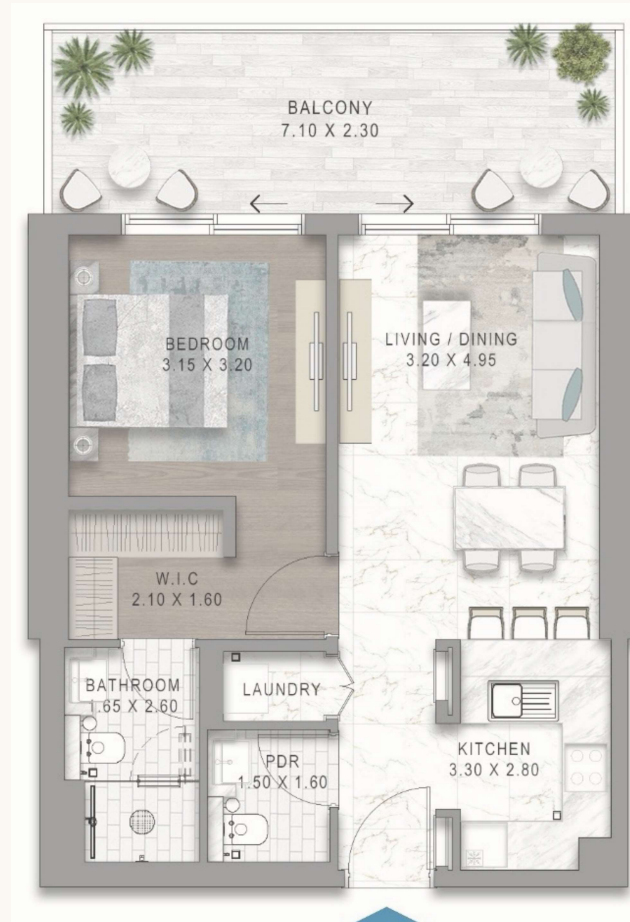
TYPE A1
